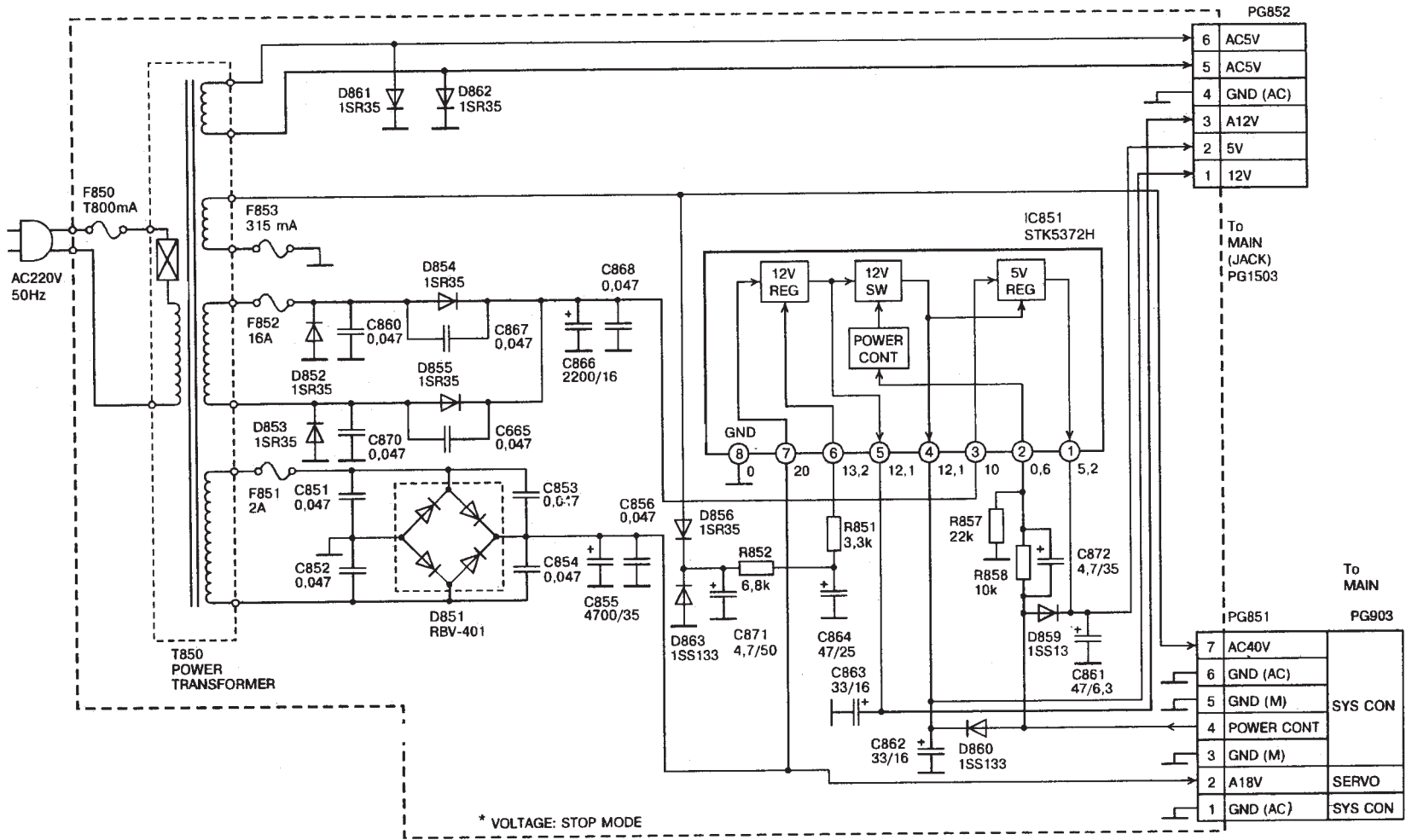
Принципиальная схема источника питания видеомагнитофонов VT-416E/400E/410E/425E
